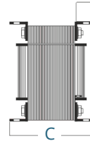
E-I Tipi Saclı Reaktör
